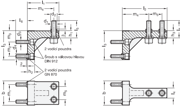
Příklady montáže
